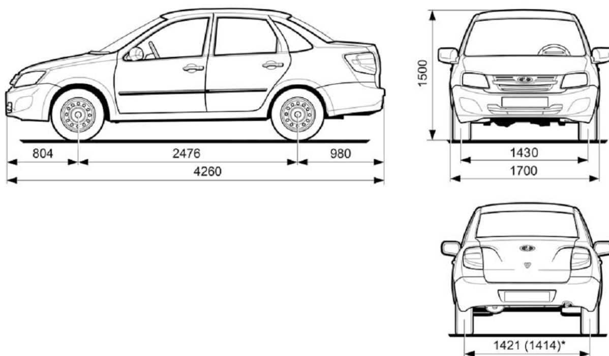
Рис. 1. Основные размеры автомобиля ВАЗ 2190 Lada Granta
