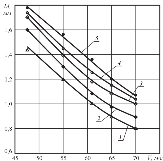
Рис. 2. Зависимость модуля помола от окружной скорости молотков:
