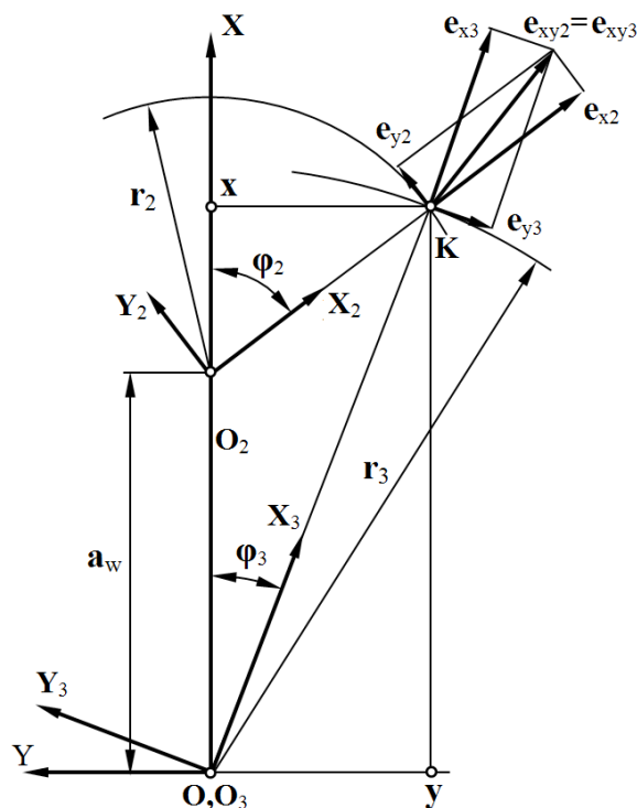
Рис. 4. Проекция точки контакта K винтовых поверхностей ролика и гайки на плоскость, перпендикулярную оси гайки: a_w – межосевое расстояние передачи
