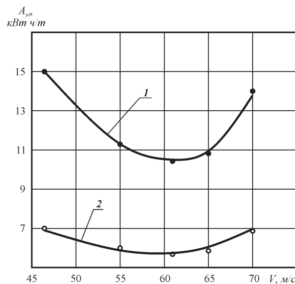
Рис. 3. Зависимости удельного расхода энергии от окружной скорости молотков: 1 – удельные затраты энергии дробилки с холостым ходом; 2 – удельные затраты энергии без холостого хода
