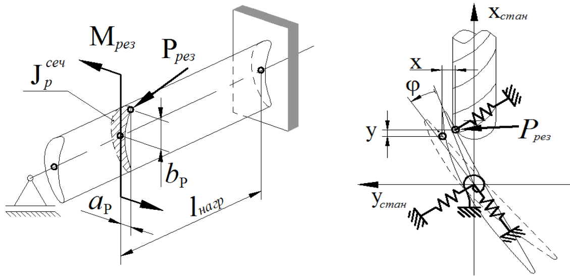
Рис. 1. Расчетная силовая схема лопатки при обработке
