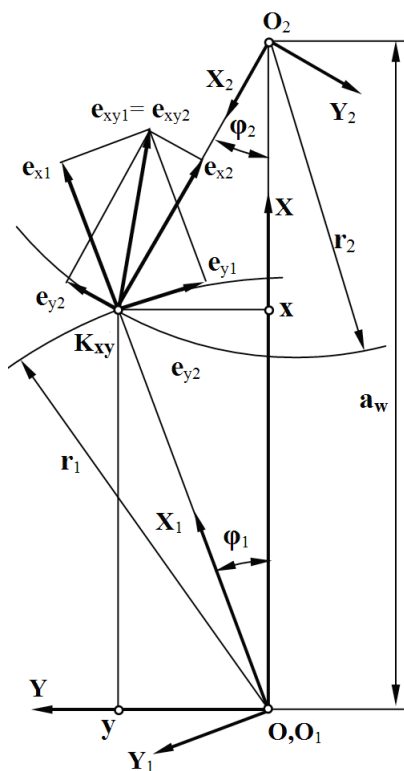
Рис. 3. Проекция точки контакта K винтовых поверхностей винта и ролика на плоскость, перпендикулярную оси винта: a_w – межосевое расстояние передачи
