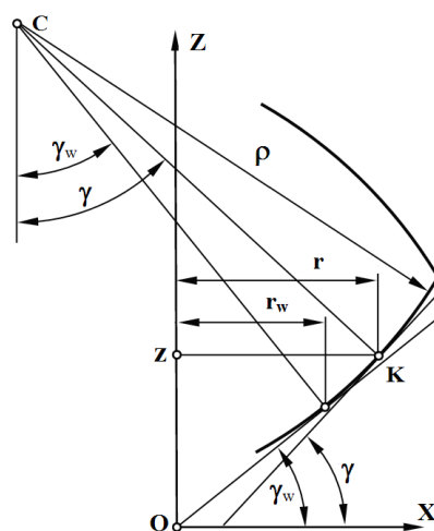
Рис. 2. Осевой профиль резьбы, модифицированный дугой окружности: \rho – радиус профилирующей окружности; r_w – радиус начальной окружности; \gamma_w – угол наклона боковой стороны профиля на начальной окружности; \gamma – угол наклона боковой стороны профиля на окружности радиуса r
