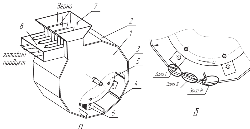
Рис. 1. Конструктивная схема безрешетной молотковой дробилки:
