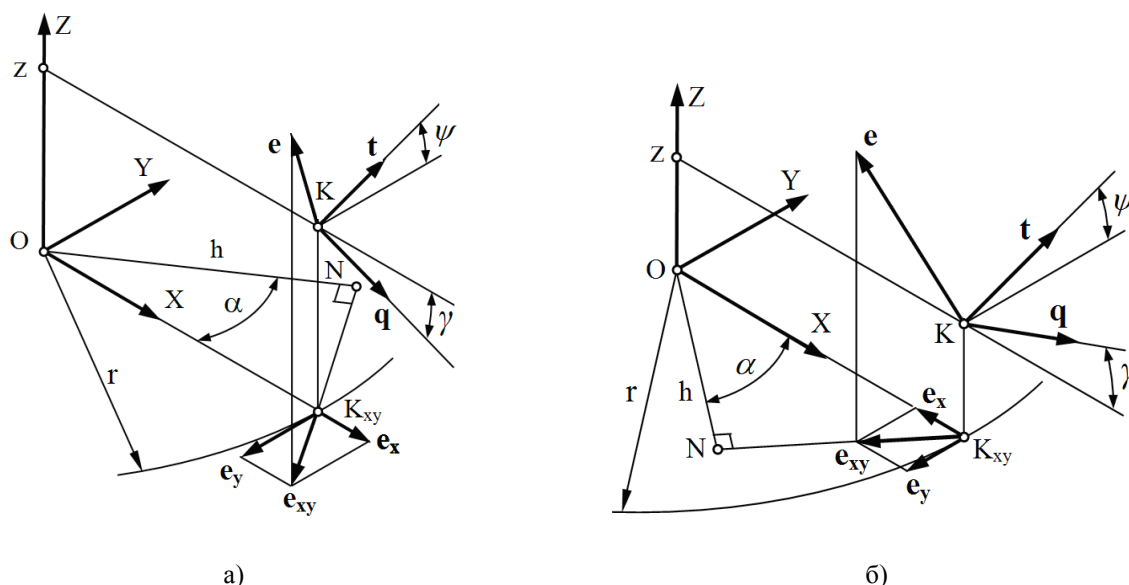
Рис. 1. Орт нормали в точке K правой винтовой поверхности в системе координат, жестко связанной с точкой K : а) верхняя сторона наружной винтовой поверхности или нижняя сторона внутренней винтовой поверхности; б) нижняя сторона наружной винтовой поверхности или верхняя сторона внутренней винтовой поверхности: ось OZ совпадает с осью винтовой поверхности, точка K лежит в плоскости XOZ ; q – орт касательной к осевому профилю поверхности; t – орт касательной к винтовой линии поверхности; \gamma – угол наклона осевого профиля; \psi – угол подъема винтовой линии поверхности на радиусе r ; \alpha – угол профиля; h – плечо профильной нормали
