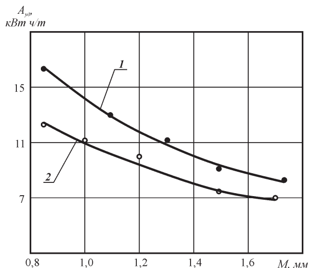
Рис. 4. Зависимость удельного расхода электроэнергии от модуля помола: 1 – серийная безрешетчатая молотковая дробилка ДБ-5; 2 – экспериментальная безрешетчатая молотковая дробилка
