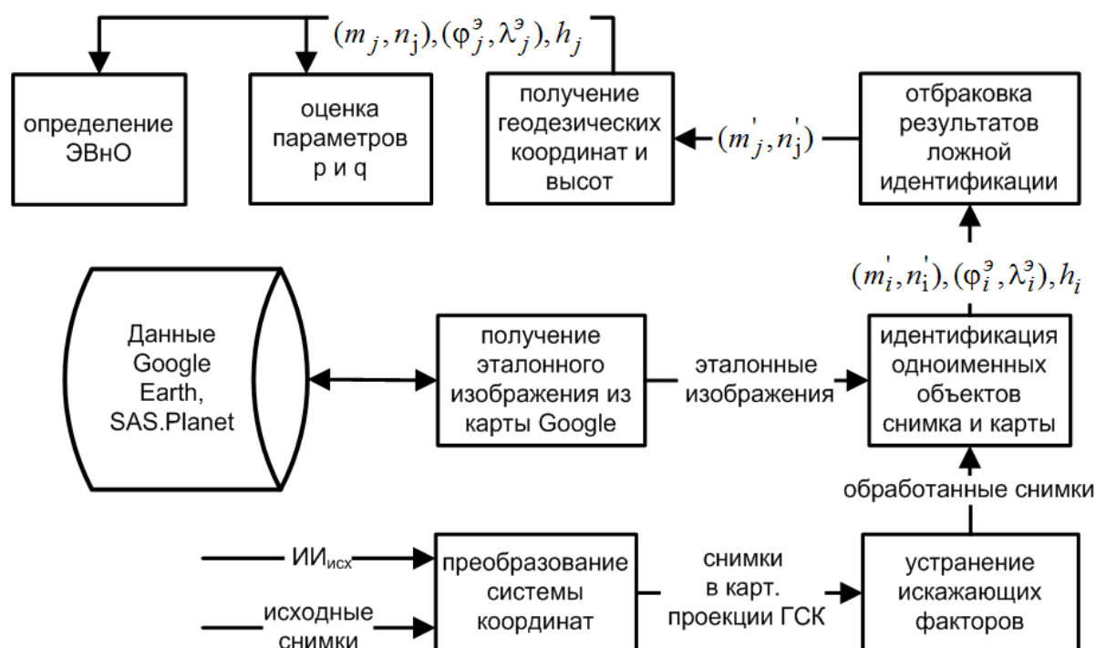
Рис. 1. Общая технология идентификации точек на изображениях с СА среднего разрешения
