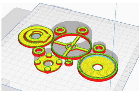
Рис. 10. Визуализация деталей колесного редуктора в Ultimaker Cura
