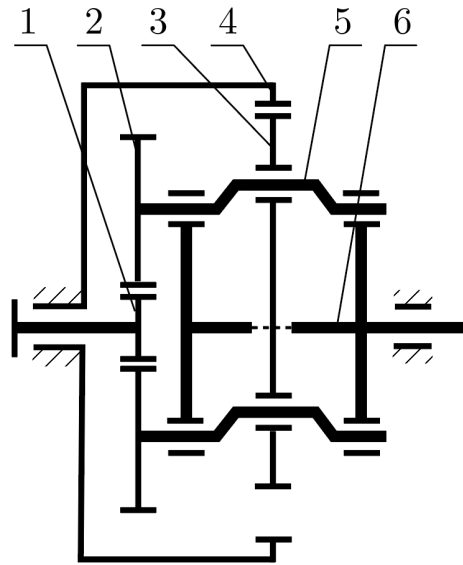
Рис. 1. Планетарно-цевочный редуктор по схеме 2K-V: 1 – солнечная шестерня; 2 – сателлит эвольвентной ступени; 3 – сателлит циклоидальной ступени; 4 – обойма с цевками; 5 – эксцентрик; 6 – выходной вал
