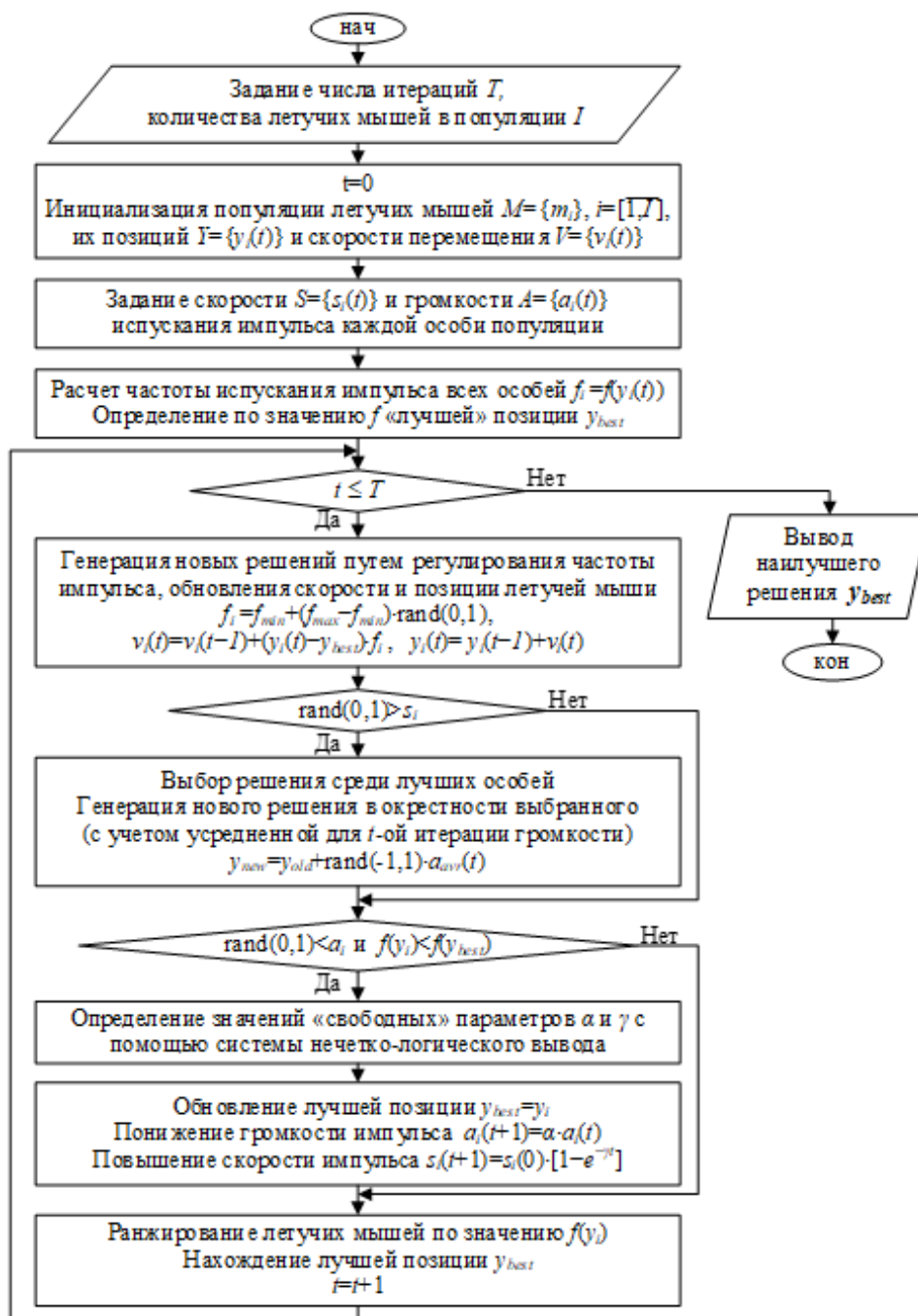
Рис. 3. Блок-схема модифицированного ВА-алгоритма
