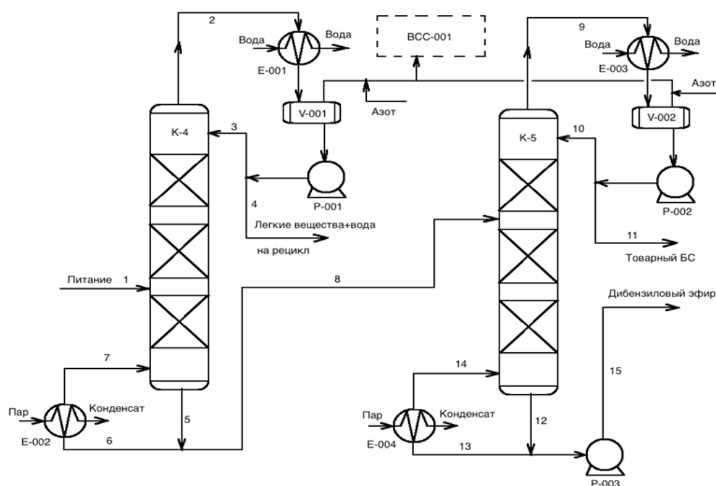
Рис. 2. Принципиальная технологическая схема выделения бензилового спирта из продуктов гидролиза бензилхлорида. E-001–004 – теплообменники; V-001–002 – емкости; P-001–003 – насосы; BCC-001 – вакуум-создающая система
