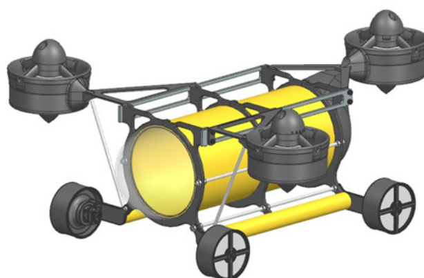
Рис. 4. Внешний вид разработанной конструкции
