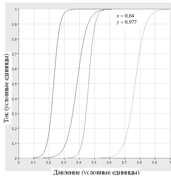
Рис. 5. Характеристики пьезорезистивных такселов с различными наполнителями
