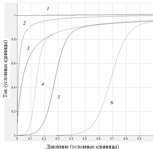
Рис. 6. Характеристики такселей с различными механизмами проводимости: 1 – объемная проводимость; 2–3 – проводимость при наличии зазоров в контакте; 4–6 – проводимость при наличии перколяционных механизмов
