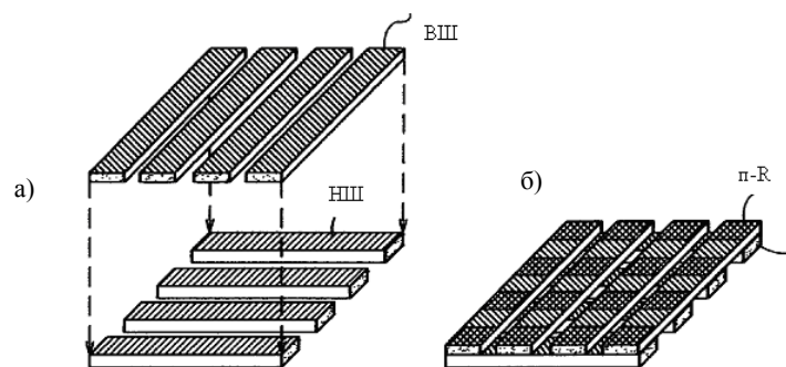
Рис. 1. Простейшая архитектура Т-сенсора
