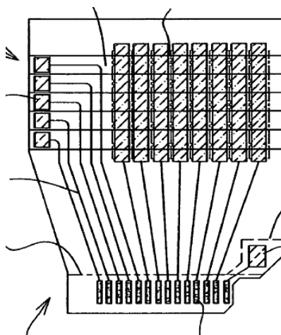
Рис. 2. Т-сенсор на гибкой подложке
