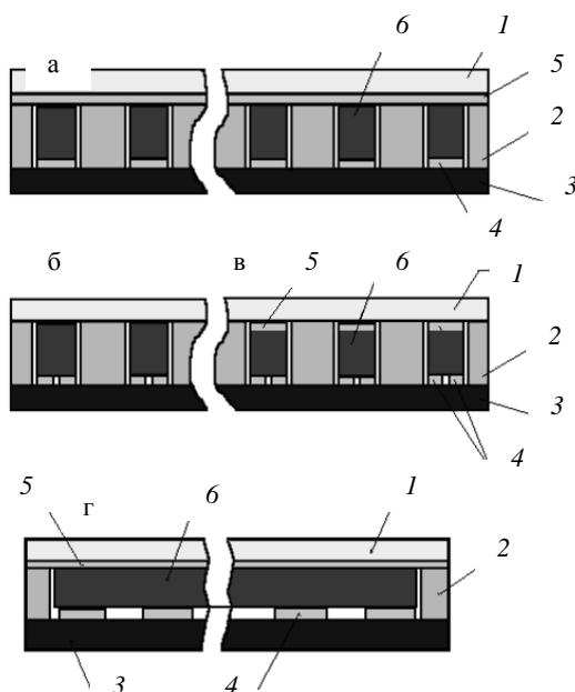
Рис. 3. Варианты конструкции такселов:
