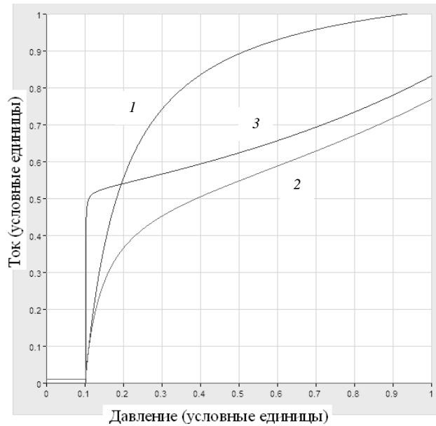
Рис. 4. Варианты характеристики объемно-контактного таксела: 1 – при определяющей роли контактного сопротивления; 2 – при наличии шероховатости поверхности; 3 – при определяющей роли объемного сопротивления
