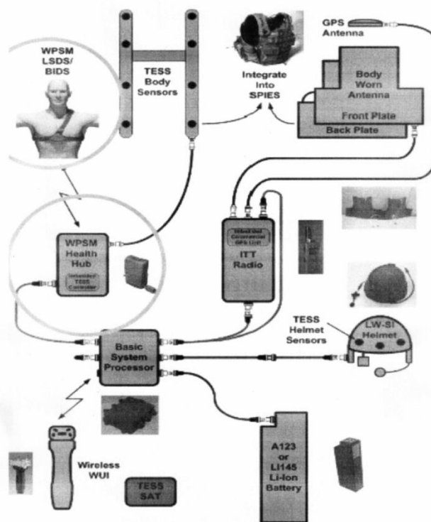
Рис. 2. Единая электронная система, объединяющая БМ с другими функциями системы FFW
