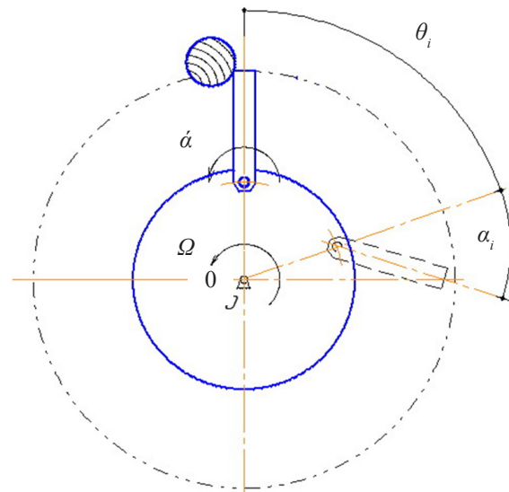
Рис. 1. Расчетная схема встречи ножа с древесным стволом:
