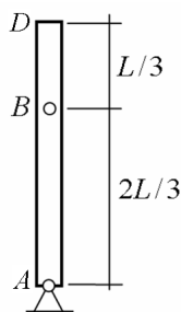
Рис. 2. Центр удара в точке B
