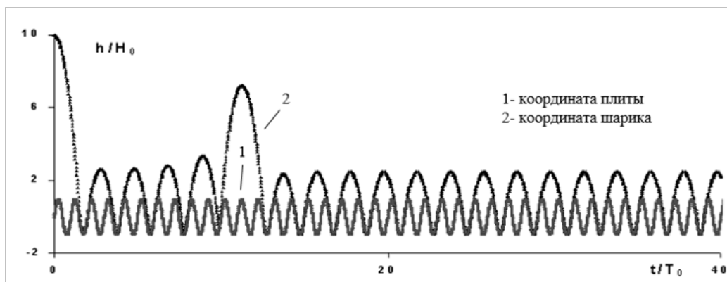
Рис. 1а. Временная зависимость расстояния шарика h до начального положения плиты в нормированных координатах при значениях параметров: g = 10 \text{ м/с}^2 , H_0 = 0,3 \text{ м} , w = 4\pi \text{ с}^{-1} , T_0 = 2\pi/w , R^* = 0,61 , R = 0,6
