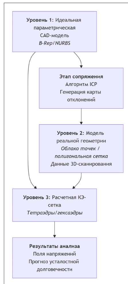
Рис. 1. Схема построения иерархической геометрической основы цифрового двойника для задач прочности
