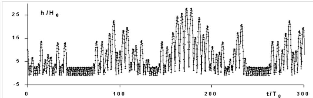
Рис. 2а. Временная зависимость h(t) для R = 0,62 при критическом R^* = 0,61
