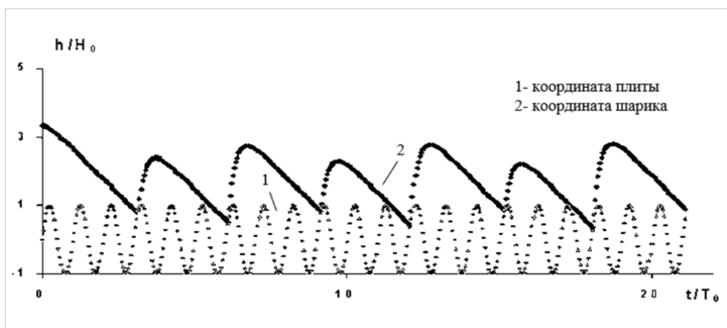
Рис. 1б. Временная зависимость расстояния шарика h до начального положения плиты в нормированных координатах при значениях параметров: g = 10 \text{ м/с}^2 , H_0 = 1,0 \text{ м} , w = 6\pi \text{ с}^{-1} , B^* = 1,227 , B = 1,25
