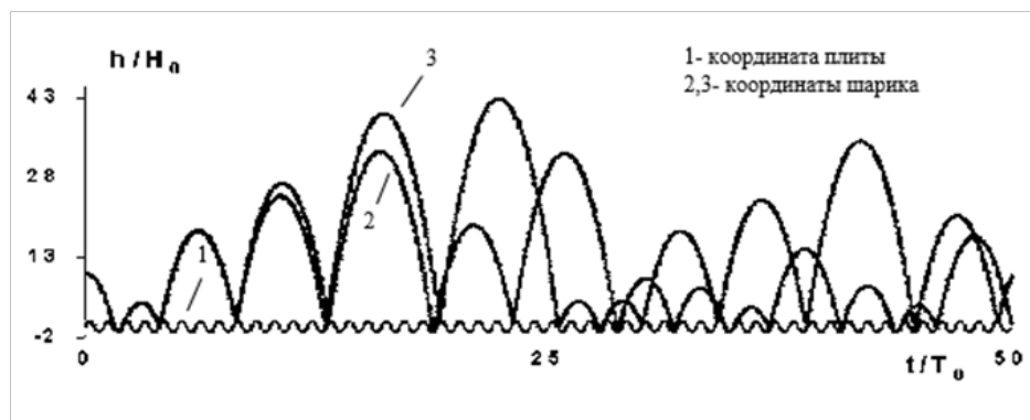
Рис. 3. Две временные зависимости h(t) , вычисленные при различных начальных высотах шарика, отличающихся менее чем на 1 %
