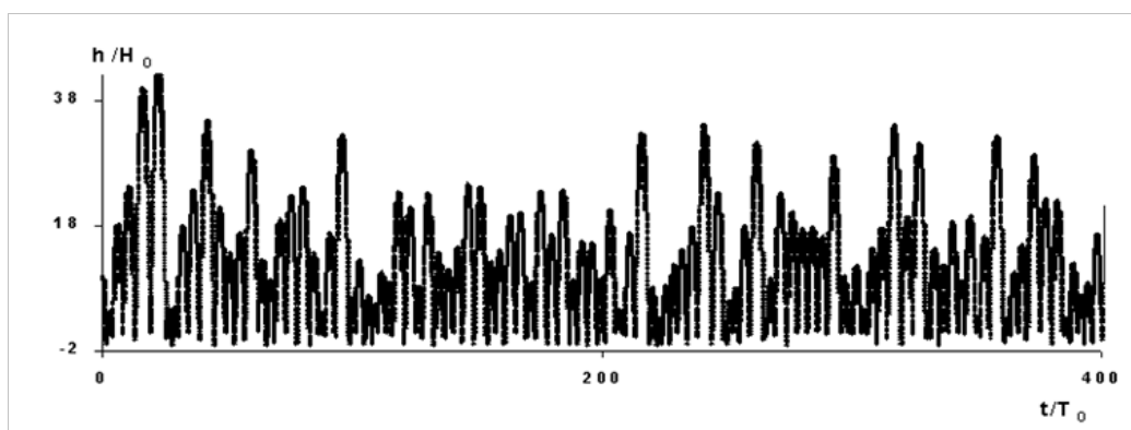
Рис. 2б. Временная зависимость h(t) для режима детерминированного хаоса при R = 0,75 при критическом R^* = 0,61
