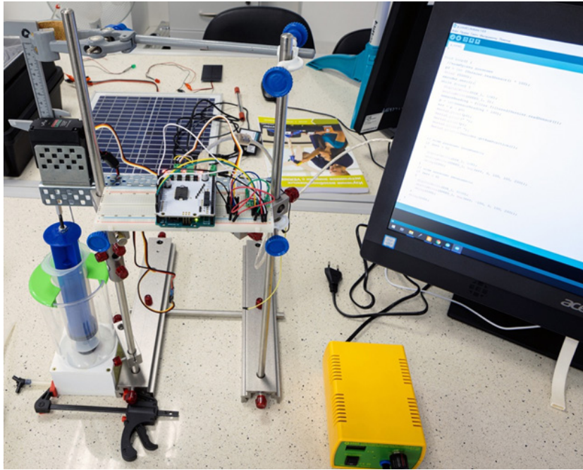
Рис. 1. Экспериментальная установка для изучения газовых законов
